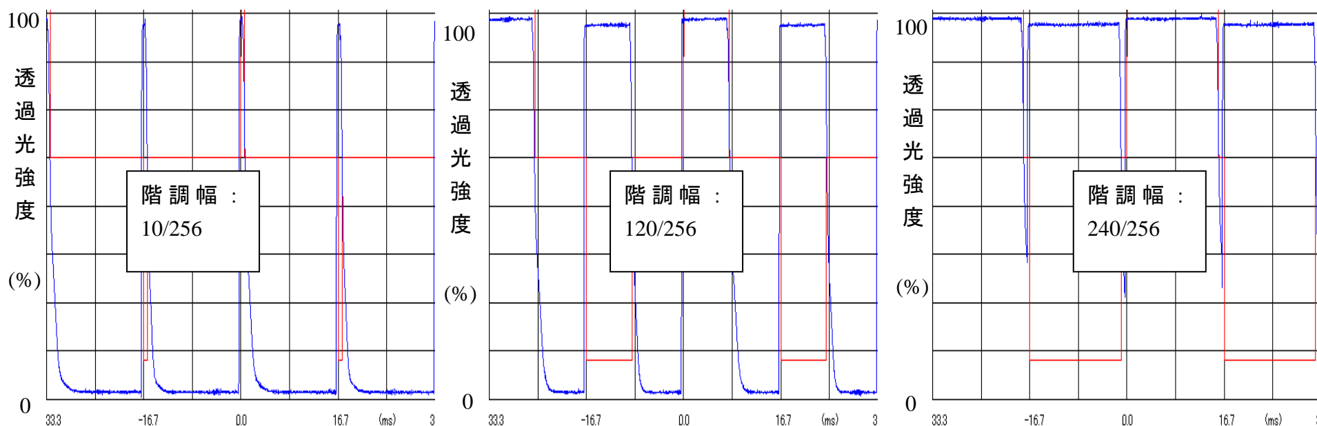
スタティック駆動での階調特性の実測図 (駆動周波数 60Hz)
